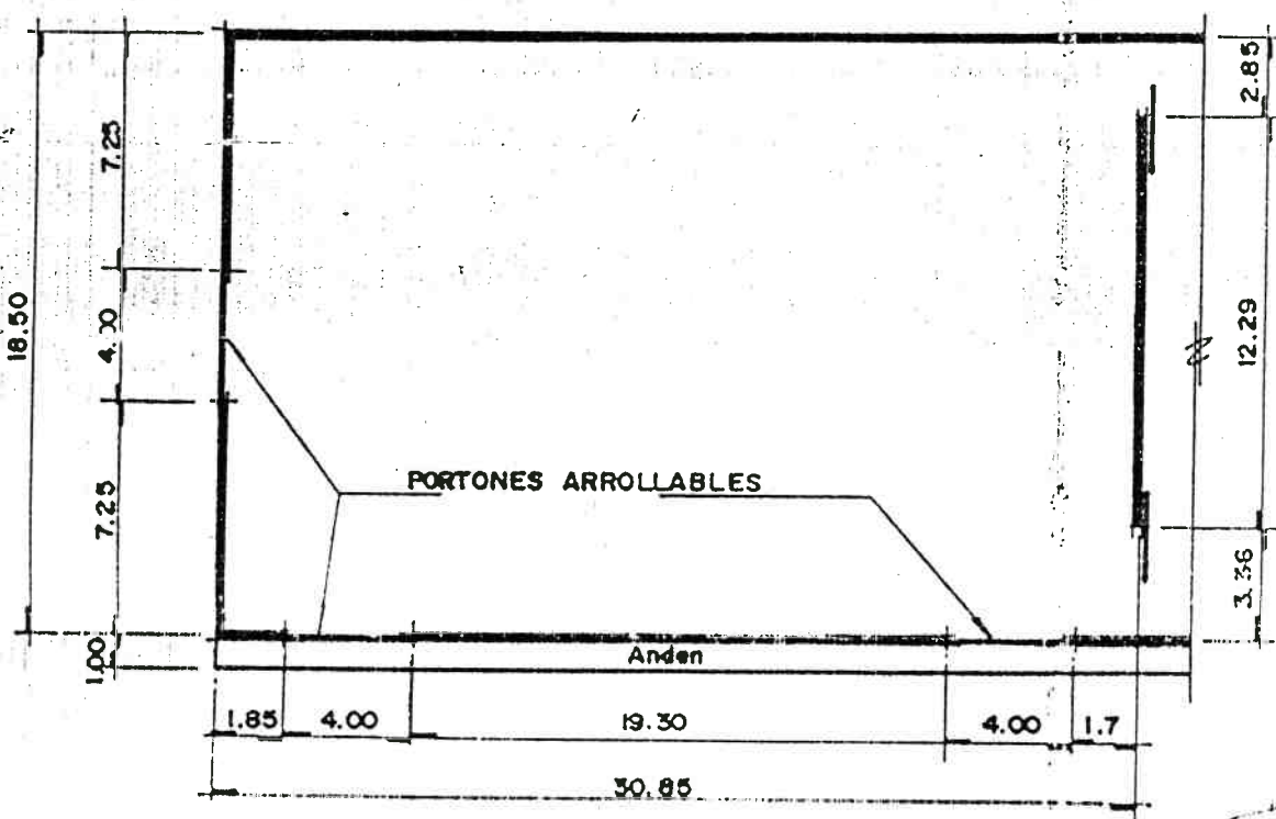
BODEGA DE ALMACENAMIENTO, CONTIGUO A PLANTA I ESC. 1:250
